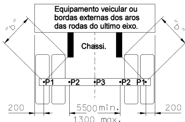
Figura A.6 – Vista traseira com cotas do ponto de aplicação
