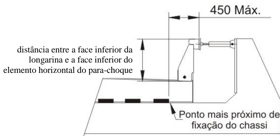
Figura A.4 – Exemplo de dispositivo de ensaio - Vista lateral
